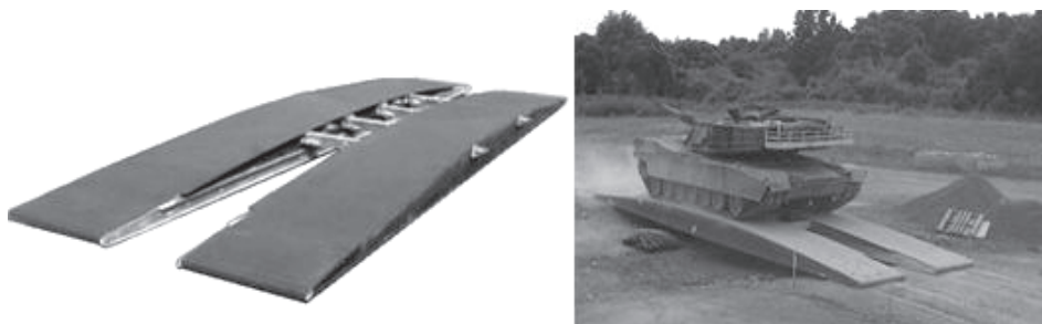
Rys. 2. Widok przęsła mostu kompozytowego CAB oraz most podczas prób zmęczeniowych [5]
