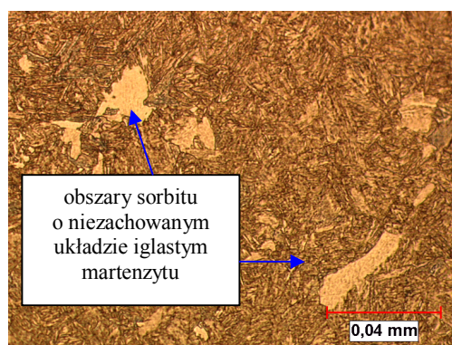
Rys. 1. Mikrostruktura badanej stali, stan trawiony, światło zwykłe, pow. 500× [13] Fig. 1. The microstructure of tested steel, etched state, conventional light, magn.500× [13]
