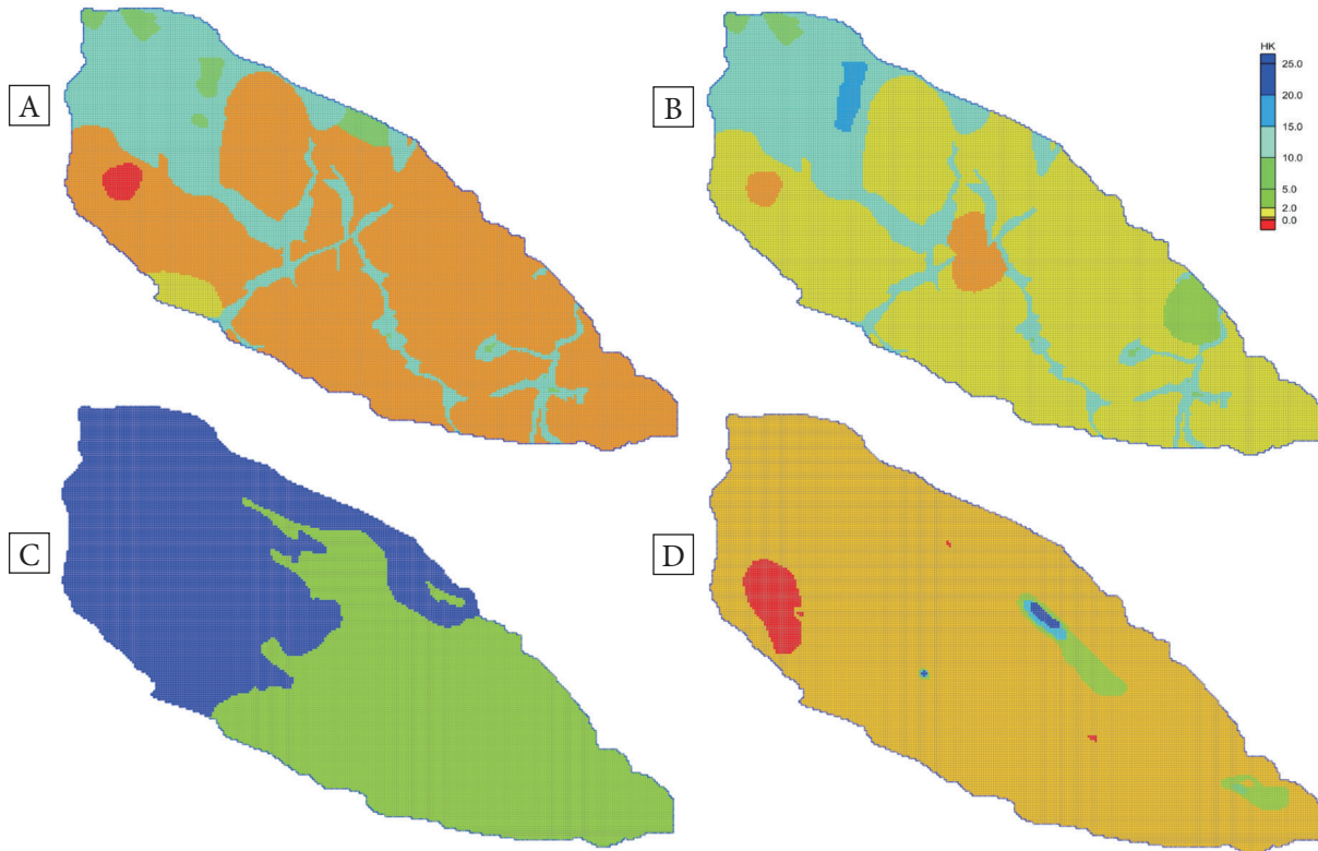
Fig. 6. Spatial distribution of hydraulic conductivity (HK in m/d) in layer 1 (A), layer 2 (B), layer 3 (C), layer 5 (D)
