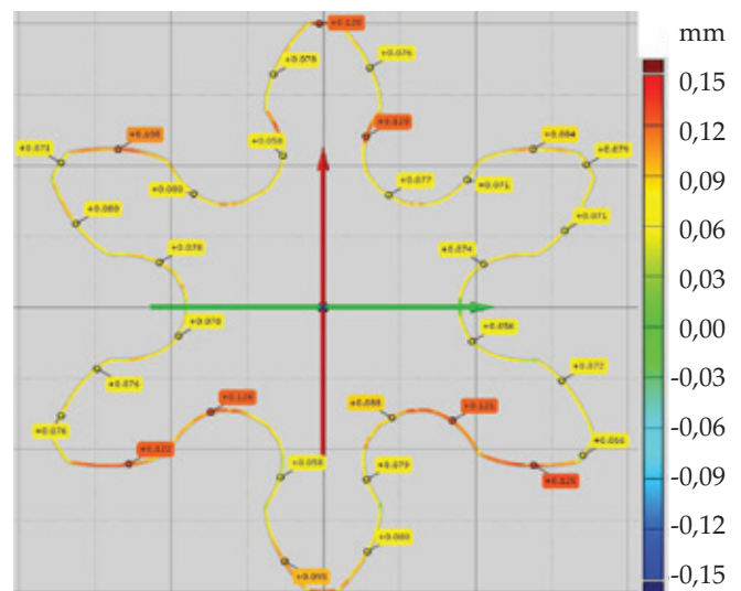
Rys. 11. Szczegółowe zestawienie odchyłek wymiarów profilu odlewu koła zębatego wytworzonego z kompozytu EPHP1IHSP3-3,0
