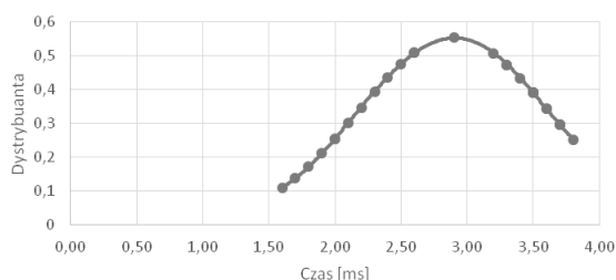
Rys. 7. Rozkład normalny czasów round-trip dla przekaźnika CB1
