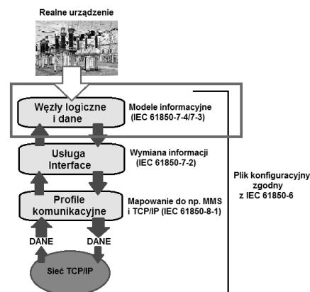
Rys. 1. Fundamentalne aspekty standardu IEC 61850
