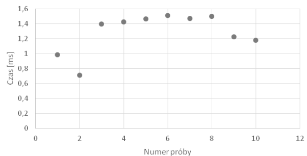
Rys. 4. Czasy GOOSE dla modelu sieci w zależności od numeru próby
