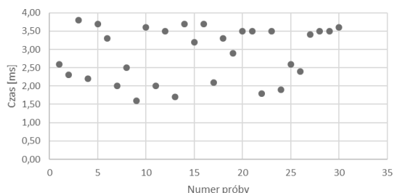
Rys. 6. Czasy round-trip dla przekaźnika CB1
