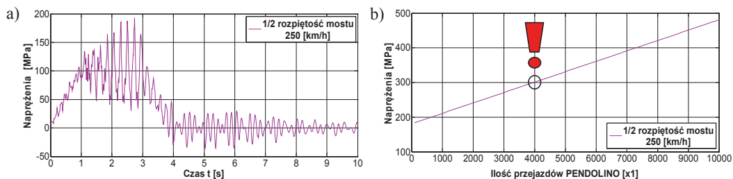
Rys. 7. Wykresy naprężeń \sigma [MPa] podczas: a) pojedynczego przejazdu, b) cyklicznego przejazdu
