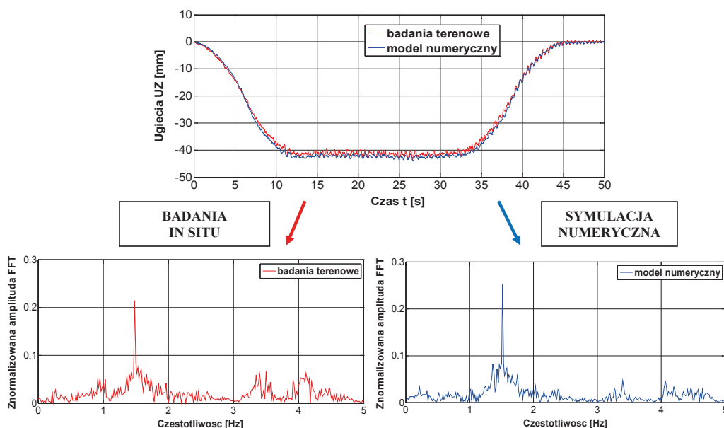
Rys. 5. Porównanie wyników ugięć w dziedzinie czasu i częstotliwości badań terenowych oraz symulacji numerycznych modelu RBT
