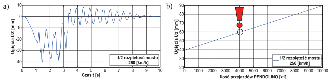
Rys. 8. Wykresy ugięcia U_z [mm] podczas: a) pojedynczego przejazdu, b) cyklicznego przejazdu
