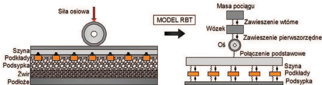
Rys. 3. Schemat zależności pomiędzy mostem-torem-tabor (pogląd empiryczny)
