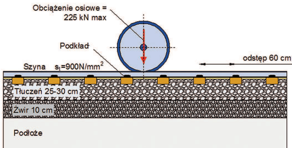
Rys. 1. Schemat i budowa toru kolejowego
