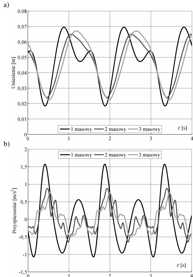
Rys. 3. Dynamika ruchu przewodu jezdnego przy różnych modelach dla v=160 \text{ km/h} , \alpha=0,29 , a) uniesienie; b) przyspieszenie
