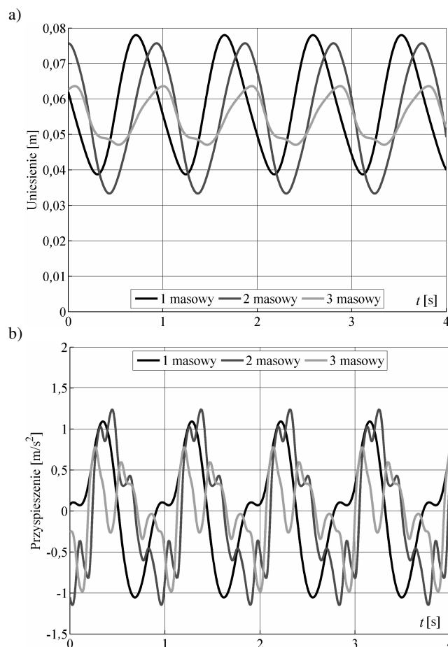
Rys. 4. Dynamika ruchu przewodu jezdnego przy różnych modelach dla v=250 \text{ km/h} , \alpha=0,17 : a) uniesienie; b) przyspieszenie
