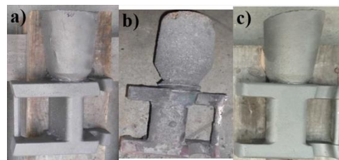
Fig. 9. Casting's variant: a) I; b) II; c) III
