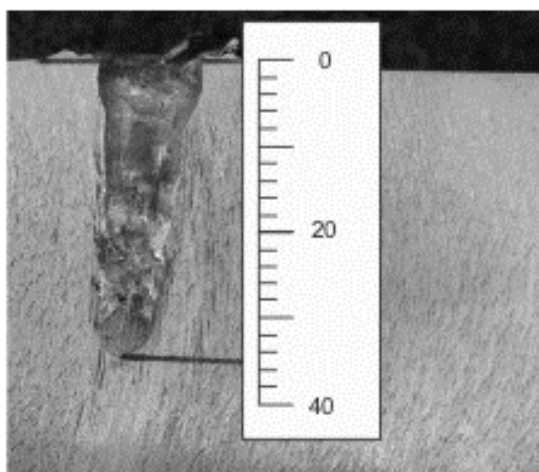
Rys. 6. Przykładowy obraz przebiccia tarczy rdzeniem badawczym
