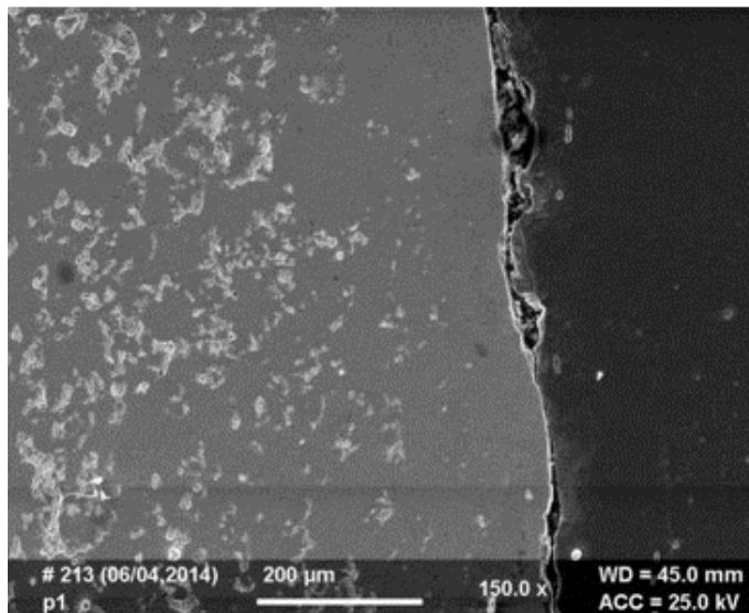
Rys. 8. Zdjęcie części wierzchołkowej rdzenia, pow. 150x
