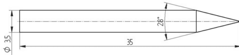
Rys. 2. Wymiary rdzeni pocisków doświadczalnych zastosowanych w badaniach
