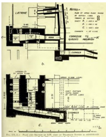
Rys.1. rzut i przekrój systemu kanalizacyjnego Południowo – zachodniej części Pałacu w Knossos; [10]
