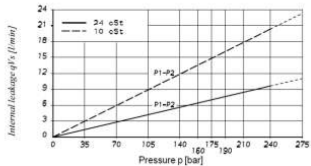
Rys. 3.2 Zależność strumienia strat wolumetrycznych związanych z przeciekami między elementami roboczymi pompy od ciśnienia roboczego pompy [13]
