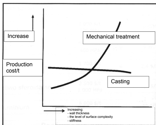
Rys. 3. Schemat ogólne porównania kosztów elementu odlewniczego i wykonanego przez obróbkę mechaniczną Fig. 3. General scheme of the comparison of the costs of cast element and element made by machining
