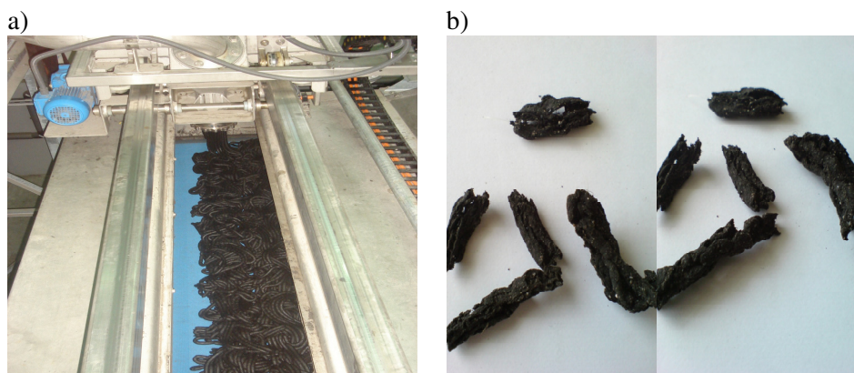
Rys. 1. Osad ściekowy: a) dozowany na górną taśmę przenośnika suszarni, b) wysuszony osad ściekowy o zawartości 90% suchej masy [6] Fig. 1. Osad a sewer: a) sludge dispensed on top of a conveyor belt dryer, b) the dried sludge with a content of 90% dry matter [6]
