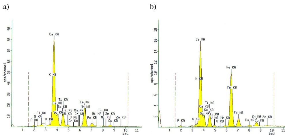
Rys.2. Analiza intensywności fluoroscencyjnych linii widmowych przy analizie energodispersyjnej wysuszonego osadu ściekowego: a) przed spopieleniem, b) po spopieleniu [badania własne]
