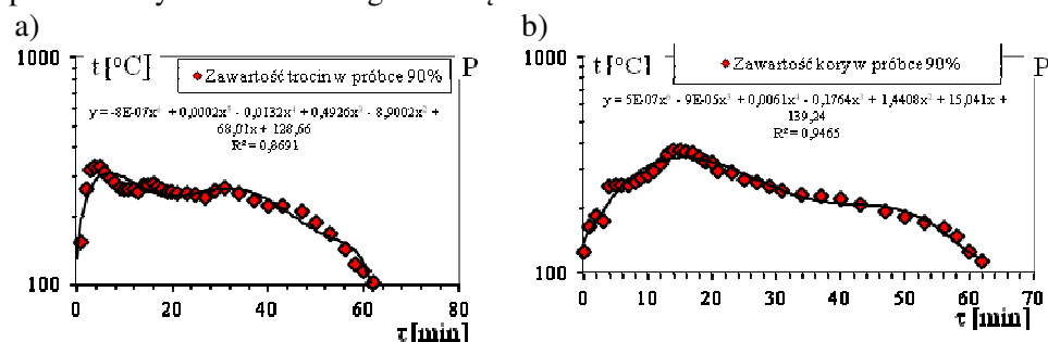
Rys. 3. Zmiany temperatury przy współpalaniu wysuszonego osadu ściekowego o zawartości 90% suchej masy z: a) trocinami, b) kora sosnową [badania własne]
