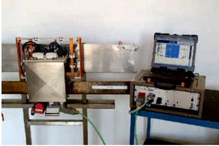
Rys. 24. Widok skanera Phased-Array w trakcie kalibracji na bloku referencyjnym
