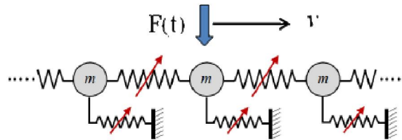
Rys. 1. Model układu z ruchomym obciążeniem Fig. 1. Model of system with moving load
