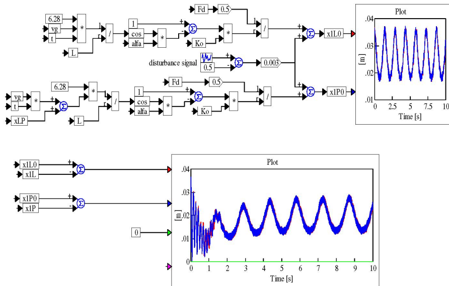
Rys.8. Schemat blokowy części głównej programu symulacji, która służy do symulacji ugięć drutu jezdny, zarówno statycznych x_{IL0} , x_{IP0} , jak i przemieszczeń zmiennych w czasie x_{IL}(t) , x_{IP}(t) w punktach kontaktu ślizgaczy z drutem jezdny; uwzględniono losowy charakter zakłóceń w postaci szumu białego Fig.8. Block diagram of the main part of VisSim program of simulation of wire displacements: x_{IL0} , x_{IP0} (static) and also x_{IL}(t) , x_{IP}(t) of the active pantograph model, it was taken into consideration random disturbances in form of white noise
