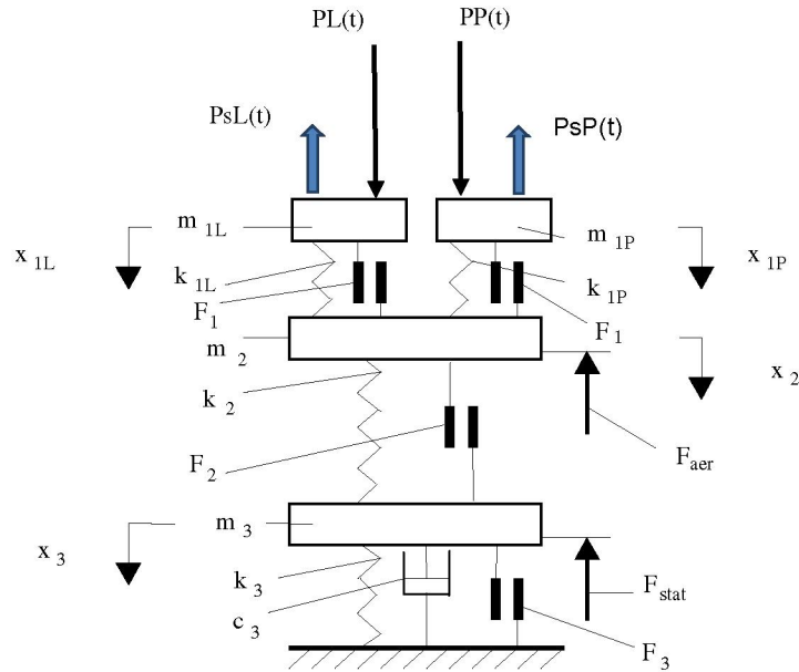
Rys. 4. Model aktywnie sterowanego odbieraka prądu; składowe siły PsL(t) i PsP(t) są realizowane poprzez aktywatory i wpływają na wypadkowe siły docisku PL(t) i PP(t) ślizgaczy do przewodu jezdnego
