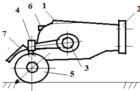
Рисунок 11. Симметричная конструкция трактора из двух тягово-приводных электромодулей. Обозначения: 1 – корпус с электронакопителем; 2 – стыковочный узел; 3 – подпружиненный рукав колесной опоры; 4 – поворотный приводной шарнир; 5 – ведущее поворотное колесо; 6 – ВОМ; 7 – панели солнечных батарей.
