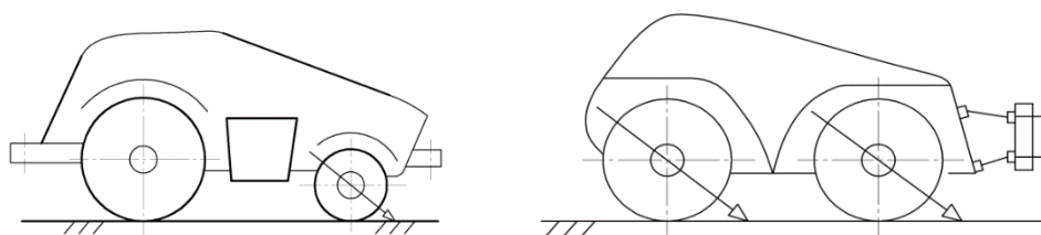
Рисунок 7. Схема беспилотного трактора 4x4 Рисунок 8. полноприводный трактор с передними и задними сцепными системами поворота типа «краб» устройствами.
