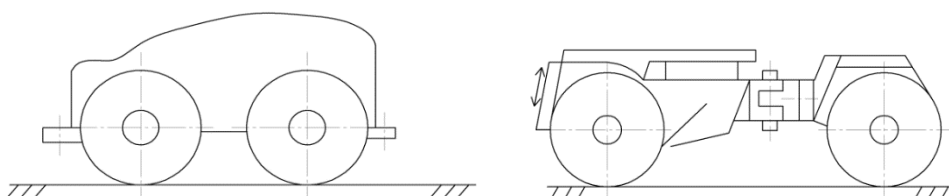
Рисунок 9. Схема беспилотного короткобазного трактора 4x4 с бортовой схемой поворота с возможностью оборудования с помощью универсальных электроуправляемых евроадаптеров. Рисунок 10. Схема мощного беспилотного полноприводного шарнирно-сочлененного трактора.
