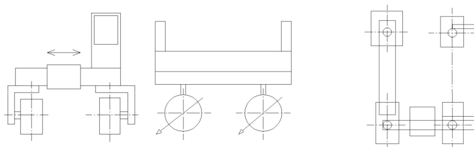
Рисунок 12. Схема приводных несущих платформ с индивидуальным гидростатическим или электроприводом колес
