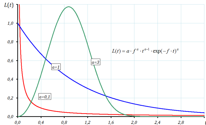
Rys. 2. Gęstość rozkładu prawdopodobieństwa L(t) rozkładu Weibulla dla różnych wartości parametru \alpha i częstości f = 1 .
