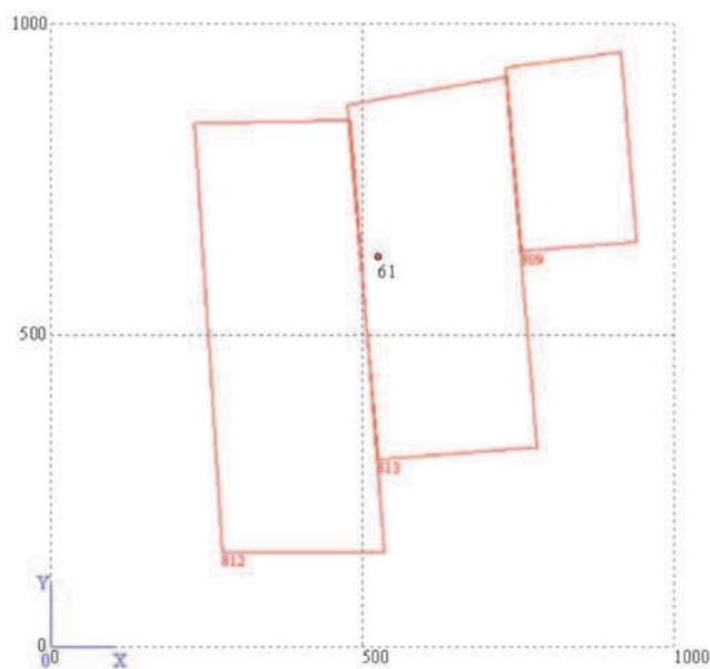
Rys. 2. Lokalizacja punktu pomiarowego względem dokonanej eksploatacji górniczej
