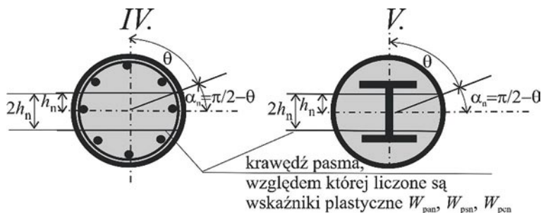
Rys. 3. Schematy geometrii analizowanych przekrojów służące do określenia wartości h_n
