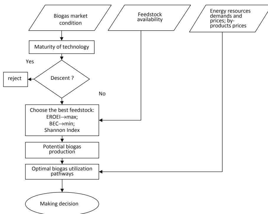
Fig. 18. Flow chart
