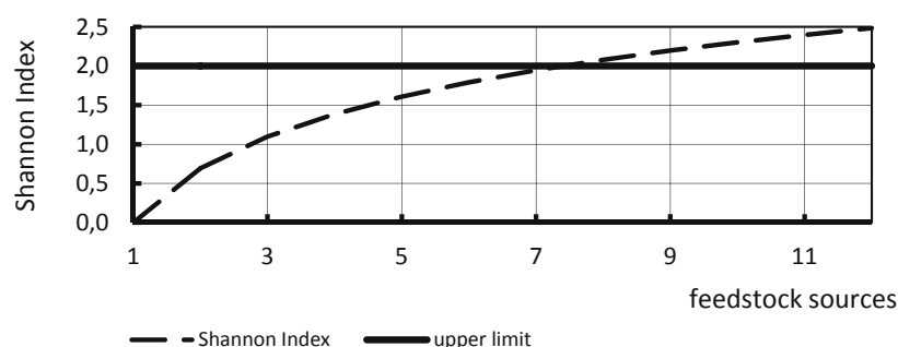
Fig. 12. Shannon Index
