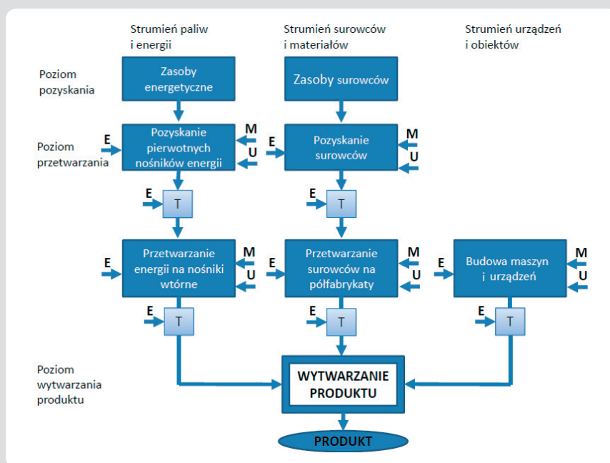
Rys. 2. Schemat ideowy do obliczeń energochłonności skumulowanej: E – energia dostarczona bezpośrednio, M, U – energia zawarta w użytych maszynach i urządzeniach, T – transport, źródło: [4, 7]
