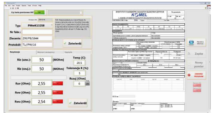
Rys. 11. Przyrząd wirtualny do badania generatorów synchronicznych z magnesami trwałymi
