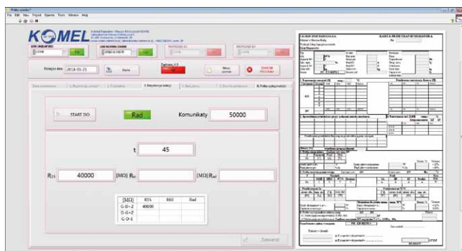
Rys. 13. Przyrząd wirtualny do badania transformatorów energetycznych
