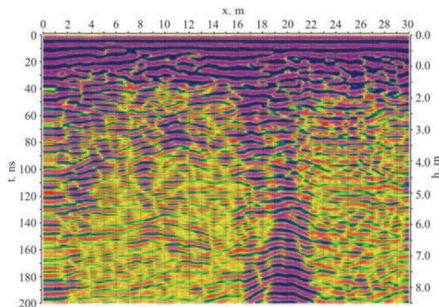
Rys. 3. Echogram pomiarowy dla profilu z zaznaczającą się strefą anomálną w postaci wzrostu amplitudy Fig. 3. Radargram of profile with anomalous zone in the form of amplitude increase
