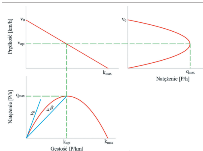
Rys. 1. Przykładowy model zależności prędkość – gęstość – natężenie z oznaczeniem punktów charakterystycznych
