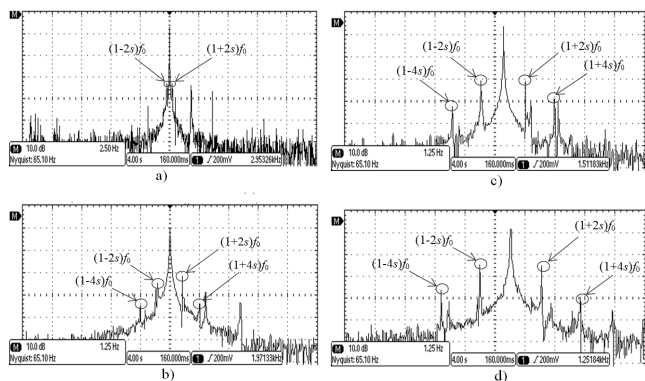
Rys. 3. Symptomy uszkodzenia w widmie prądu fazowego stojana przy znamionowej prędkości kątowej oraz momencie obciążenia (a) M_o=0 ; (b) M_o=0,3 ; (c) M_o=0,5 ; (d) M_o=0,65 [j. w.] w silniku klatkowym przy asymetrycznym wirniku
