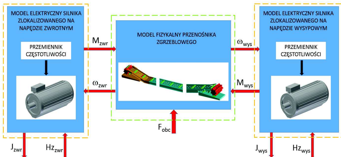
Rys. 1. Model obliczeniowy przenośnika zgrzeblowego. Model fizyczny przenośnika – przerywana linia zielona, model silników elektrycznych – przerywana linia pomarańczowa [12]
