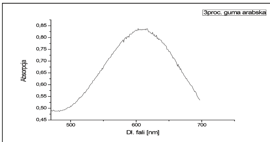
Rysunek 5. Widmo UV-Vis otrzymanych nanocząstek magnetycznych otoczonych nanozłotem i stabilizowanych 3 % r-em gumy arabskiej po 120 min.
