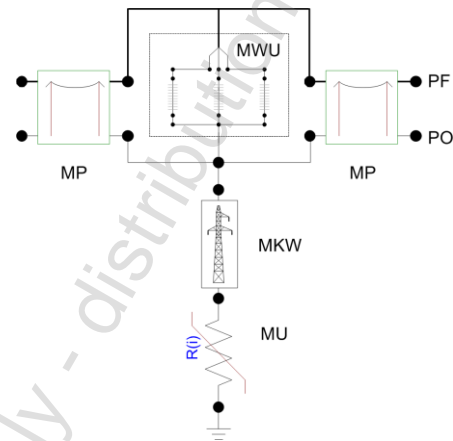
Rys. 2. Fragment modelu linii napowietrznej wykorzystany w badaniach symulacyjnych (PF – przewód fazy, PO – przewód odgromowy, MP – model przęsał, MWU – model wytrzymałości udarowej izolacji, MKW – model konstrukcji wsporczej, MU – model uziomu)
