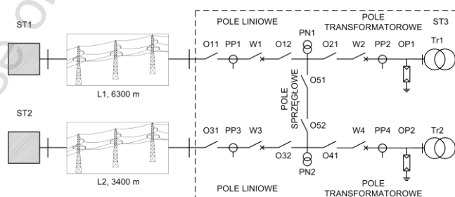
Rys. 1. Schemat rozpatrywanego układu sieci 110 kV (ST - stacja elektroenergetyczna, L - linia napowietrzna, O - odłącznik, PP - przełącznik prądowy, PN - przewodnik napięciowy, W - wyłącznik, OP - ogranicznik przepięci, Tr - transformator)
