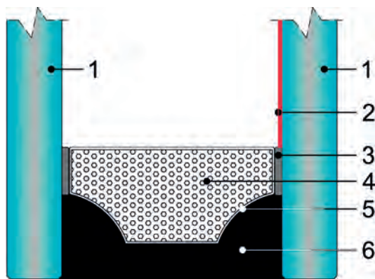
Rys. 2. Budowa szyby zespolonej:
