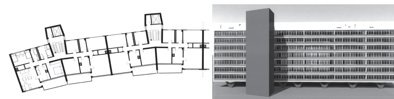
il. 5. Fragment rzutu piętra powtarzalnego, Berlin, budynek na wystawę Interbau Hansaviertel (1957), architekt Walter Gropius i The Architects Collaborative (TAC). Źródło: materiały KAWTiMP ZUT / Fragment of repetitive floor plan, Berlin, building for the Interbau Hansaviertel exhibition (1957), architect Walter Gropius and The Architects Collaborative (TAC). Source: KAWTiMP ZUT materials il. 6. Model budynku na wystawę Interbau Hansaviertel (1957), Berlin, architekt Oscar Niemeyer. Źródło: materiały KAWTiMP ZUT / Model of a building on the Interbau Hansaviertel exhibition (1957), Berlin, architect Oscar Niemeyer. Source: KAWTiMP ZUT materials
