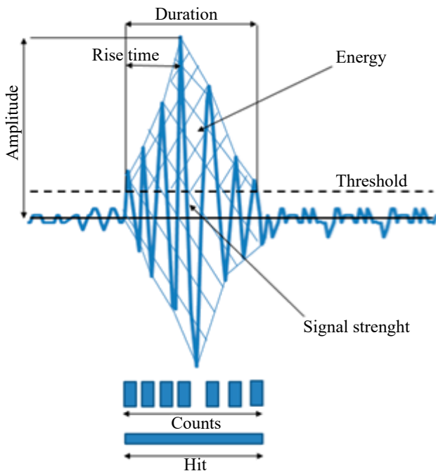
Fig. 5. Parameters reflecting of an AE waveform (ZAKI et al. , 2015).
