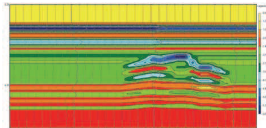
Rys. 5 Fragment syntetycznej sekcji pseudo-impedancji akustycznej generowanej dla długiego sygnału bez procedury dekonwolucji
