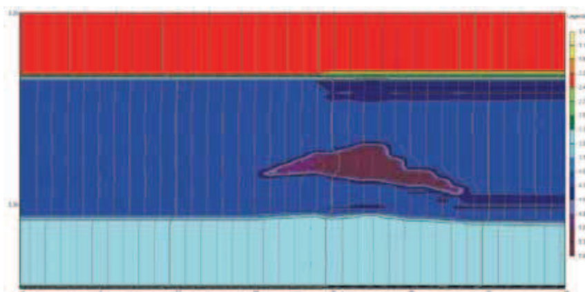
Rys. 3. Fragment syntetycznej sekcji pseudo-impedancji akustycznej generowanej dla krótkiego sygnału z wykonaną procedurą dekonwolucji minimum entropi MED Fig. 3. Fragment of the synthetic section of pseudo-acoustic impedance generated for a short signal with the minimum entropy deconvolution MED
