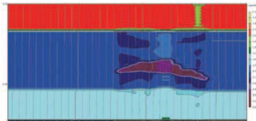
Rys. 4. Fragment syntetycznej sekcji pseudo-impedancji akustycznej generowanej dla krótkiego sygnału z wykonaną procedurą dekonwolucji predykcyjnej
