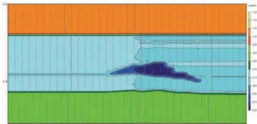
Rys. 6. Fragment syntetycznej sekcji pseudo-impedancji akustycznej generowanej dla długiego sygnału z wykonaną procedurą dekonwolucji minimum entropii MED
