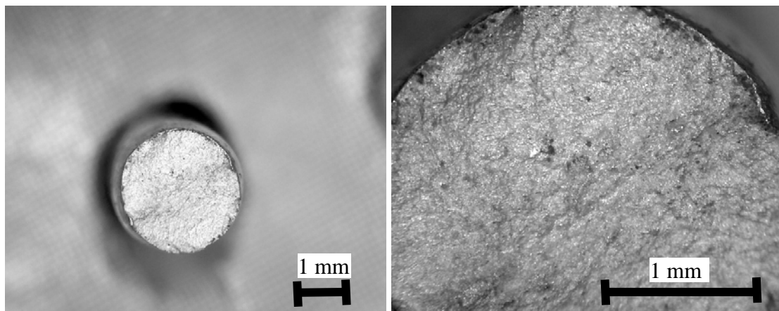
Fig. 8. Fatigue fracture of aluminum alloy containing 5% silikon for \sigma = 752.3 MPa Rys. 8. Przełom zmęczeniowy aluminium z 5% zawartością kremu dla \sigma = 752,3 MPa
