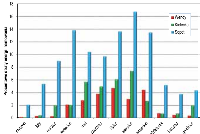
Rys. 6. Względne straty energii hamowania w skali miesięcznej w obszarach zasilania poszczególnych podstacji
