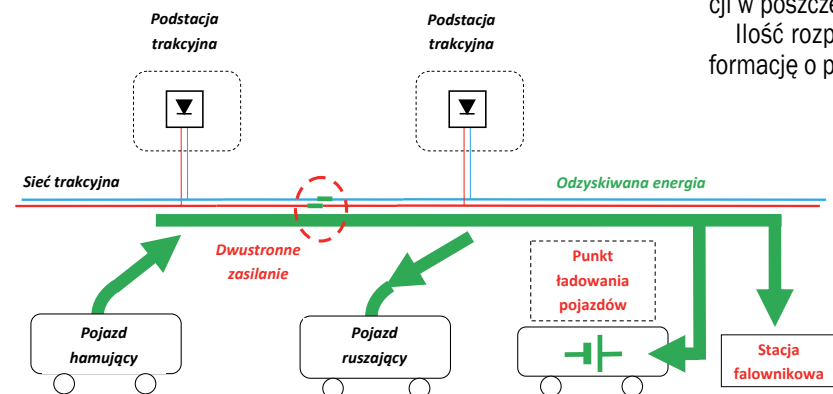
Rys. 1. Schemat przepływu energii rekuperacji z pojazdu hamującego do pojazdu ruszającego w dwustronnym układzie zasilania sieci trakcyjnej wraz ze stacją ładowania pojazdów elektrycznych oraz przekazywaniem energii odzyskanej do sieci prądu przemiennego
