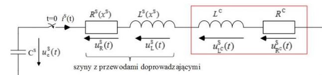
bateria kondensatorów
