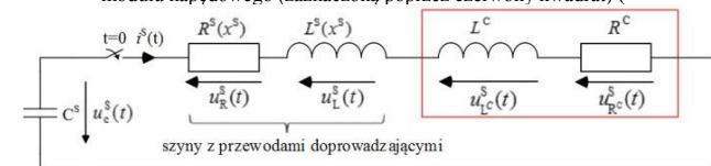
Rys. 7). bateria kondensatorów
