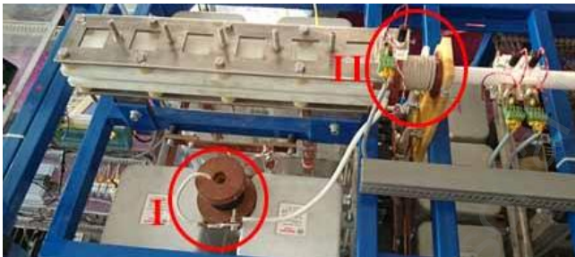
Rys. 11. Widok fragmentu hybrydowej wyrzutni elektromagnetycznej ze wspomaganie pneumatycznym, na którym elementy oznaczono następująco: I – dodatkowa cewka powietrzna, II – cewka elektromagnetycznego cewkowego modułu napędowego
