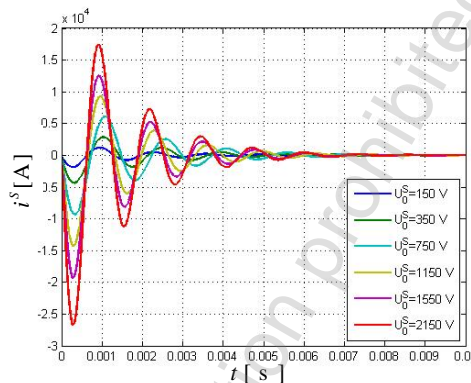
Rys. 8. Przebieg czasowy i^S = f(t) uzyskany podczas badań symulacyjnych dla elektromagnetycznego szynowego modułu napędowego – z wewnętrznym ogranicznikiem prądu (przy wartości początkowej prędkości v_0^S = 30 \frac{m}{s} )
