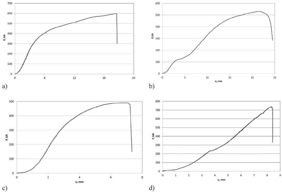
Rys. 2. Charakterystyki pracy jarzma dolnego (a) i górnego (b) strzemia SDO29, jarzma dolnego strzemia SKL (c) i jarzma dolnego strzemia SDO29w (d)
