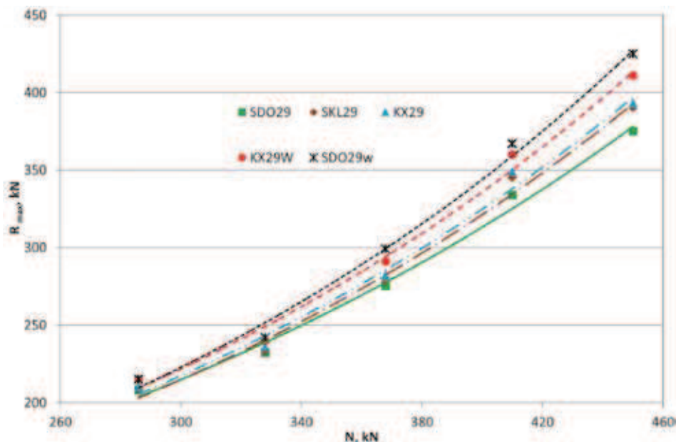
Rys. 9. Zależność maksymalnej wartości siły przenoszonej przez złącze ciernie od sumarycznej wartości wstępnych sił osiowych w śrubach strzemion dla różnych typów strzemion Fig. 9. Relationship between the maximum force conveyed by the friction joint and the total force
