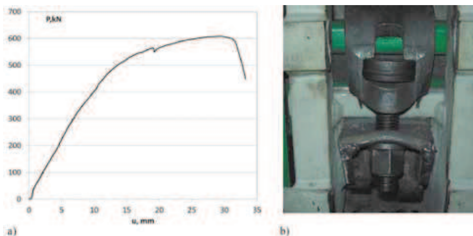
Rys. 7. Charakterystyka pracy strzemienia SDO29w (a) i jego widok po badaniu (b) Fig. 7. Characteristics of operation of the stirrup SDO29w (a) and its view after the test (b)
