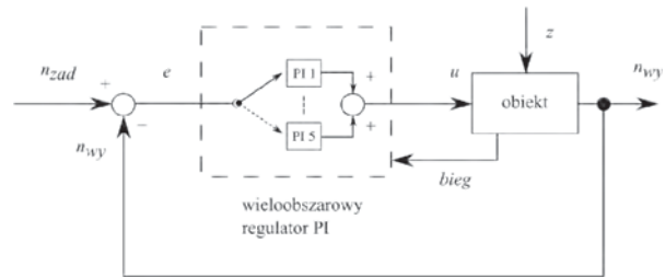
Rys. 3. Schemat wieloobszarowego układu regulacji PI Fig. 3. Scheme of multiregional PI control system
