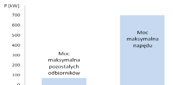
Rys. 4. Porównanie mocy maksymalnej napędu na tle mocy maksymalnej pozostałych odbiorników czerpiących energię z baterii pojazdu.
