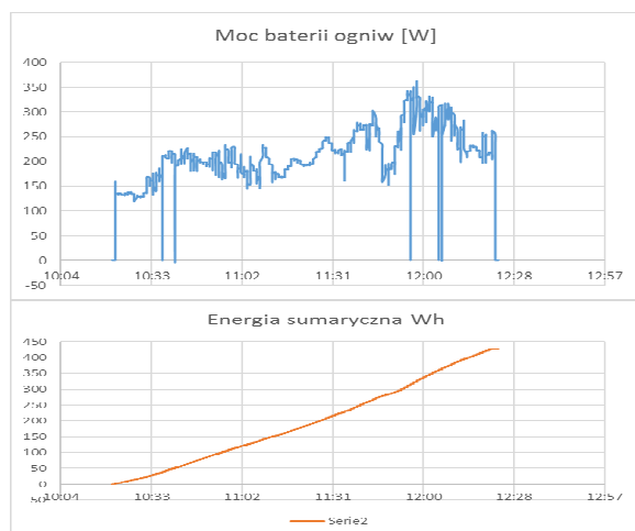
Rys. 10. Przebiegi mocy i sumarycznej energii systemu fotowoltaicznego
