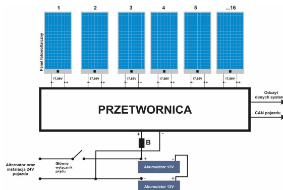
Rys. 9. Schemat blokowy pojazdowego systemu fotowoltaicznego
