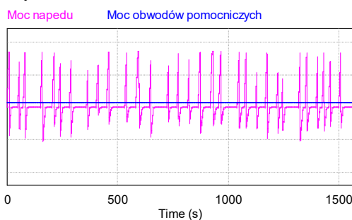
Rys. 3. Przebiegi pokazujące moc napędu na tle mocy pobieranej przez inne niż napęd urządzenia pojazdu
