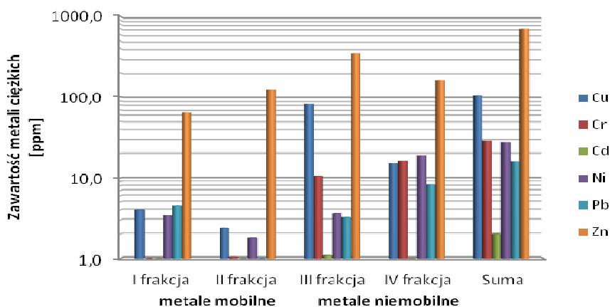
Rys. 3. Zawartość metali ciężkich w poszczególnych frakcjach uzyskanych metodą analizy specyjacyjnej
