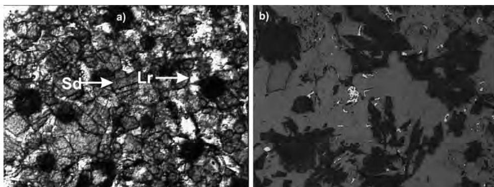
Rys. 1. Obraz mikroskopowy składników żużła hutniczego, jeden nikol, pow. 100x: a) światło przechodzące-srebrodolskit (Sd) i larnit (Lr), b) światło odbite - - jasne ziarna-stopy metaliczne w wustytowo-krzemianowym szklwie
