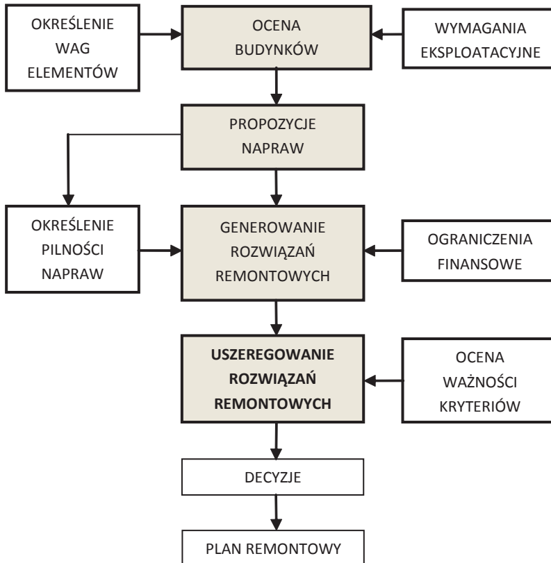
Rys. 1. Schemat proponowanej metody wyboru rozwiązania remontowego
