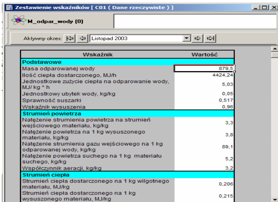
Rys. 6. Okno zestawiające wybrane wskaźniki pracy suszarki
