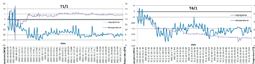
Rys. 5. Przebieg zmian naprężeń i temperatury w punkcie T1/1 zlokalizowanym na jednej z lin doprężających wezłowie oraz w T4/1 na łuku
