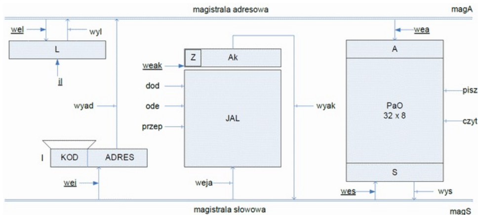
Rysunek 1. Schemat podstawowej wersji maszyny W
