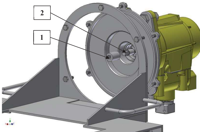
Rys. 11. Widok sprzęgła łączącego przekładnię z silnikiem pneumatycznym [3]
