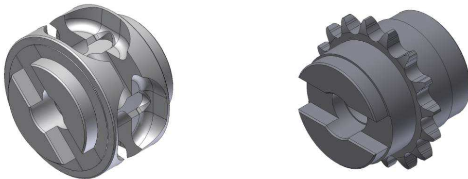
koło łańcuchowe wciągnika PWŁ 3/6
