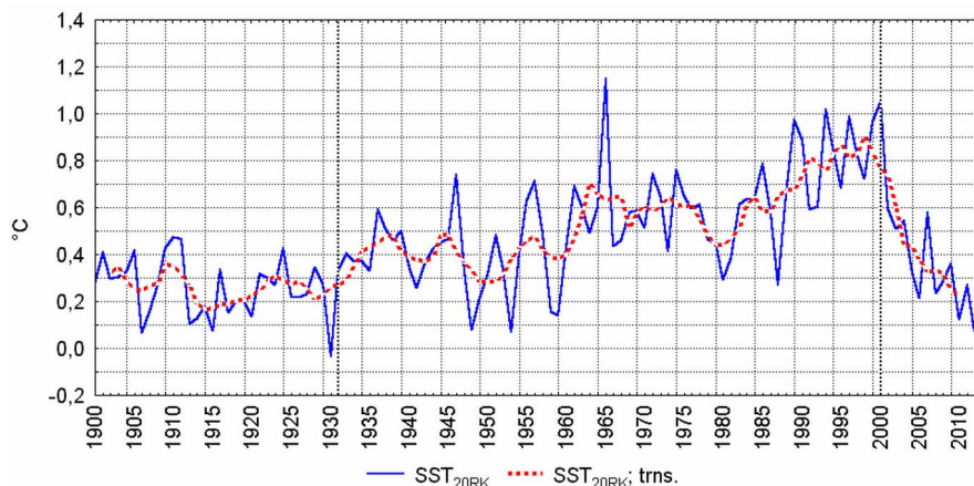
Ryc. 4. Przebieg wartości SST_{20RK} (średnia arytmetyczna z rocznych wartości w 20 gridach; patrz ryc. 2). Przebieg uśredniony – wyrównanie 5 punktową średnią konsekutywną
