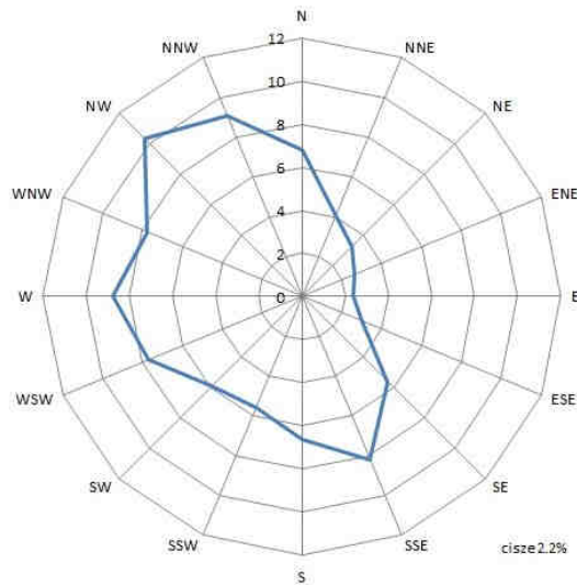
Rys. 2. Częstości kierunków wiatru na terenie Stacji Bazowej Zintegrowanego Monitoringu Środowiska Przyrodniczego Święty Krzyż w latach 2010-2014
