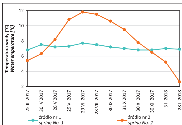
Ryc. 9. Temperatura wód źródła nr 1 i źródła nr 2 w okresie od 25.03.2017 r. do 28.02.2018 r.
