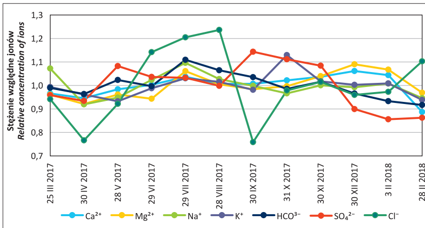
Ryc. 11. Stężenie względne jonów: \text{Ca}^{2+} , \text{Mg}^{2+} , \text{Na}^+ , \text{K}^+ , \text{HCO}_3^- , \text{SO}_4^{2-} oraz \text{Cl}^- w wodzie źródła nr 1 w okresie od 25.03.2017 r. do 28.02.2018 r.
