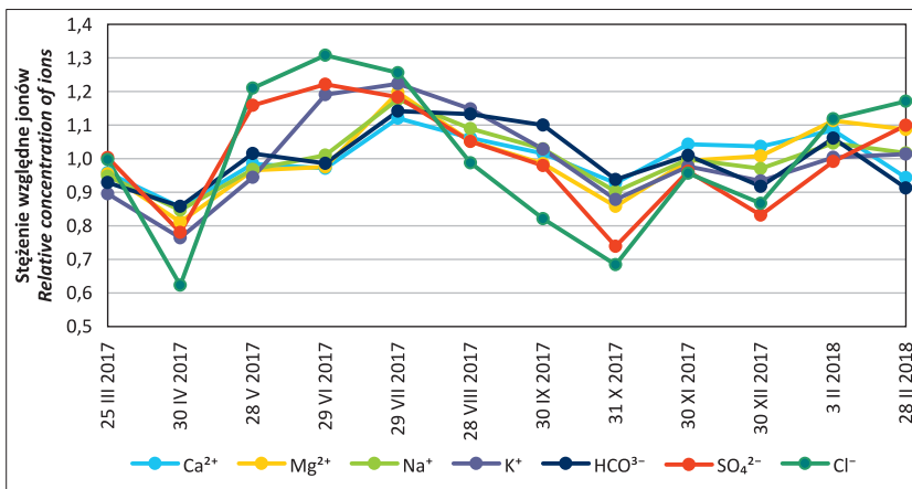
Ryc. 12. Stężenie względne jonów: \text{Ca}^{2+} , \text{Mg}^{2+} , \text{Na}^+ , \text{K}^+ , \text{HCO}_3^- , \text{SO}_4^{2-} oraz \text{Cl}^- w wodzie źródła nr 2 w okresie od 25.03.2017 r. do 28.02.2018 r.
