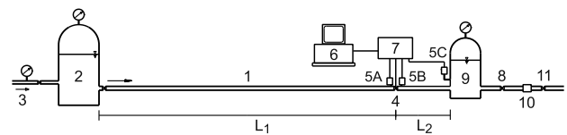
Rys 1. Schemat stanowiska pomiarowego Fig 1. Scheme of experimental setup
