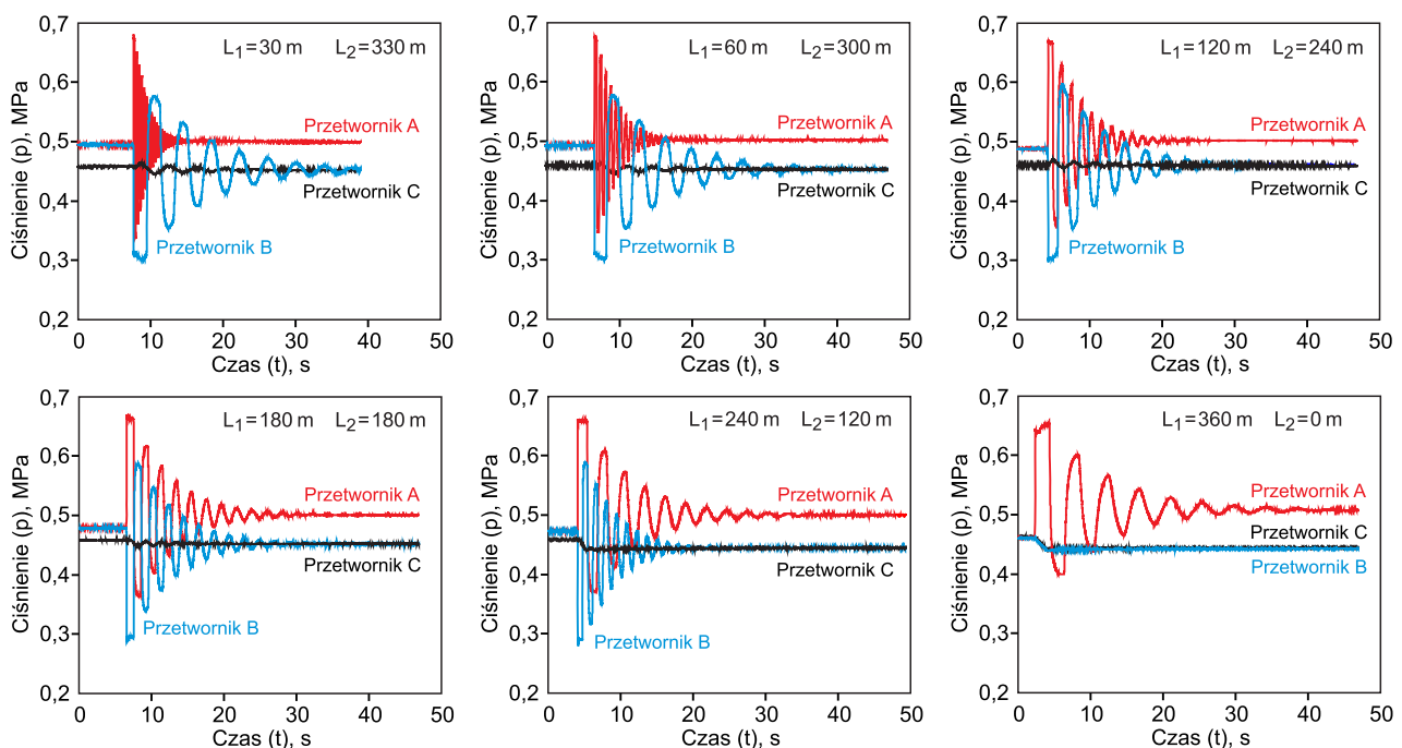
Rys. 2. Przykładowe zmierzone charakterystyki ciśnienia podczas uderzenia hydraulicznego przy prędkości przepływu wody w ruchu ustalonym równej 0,5 m/s
