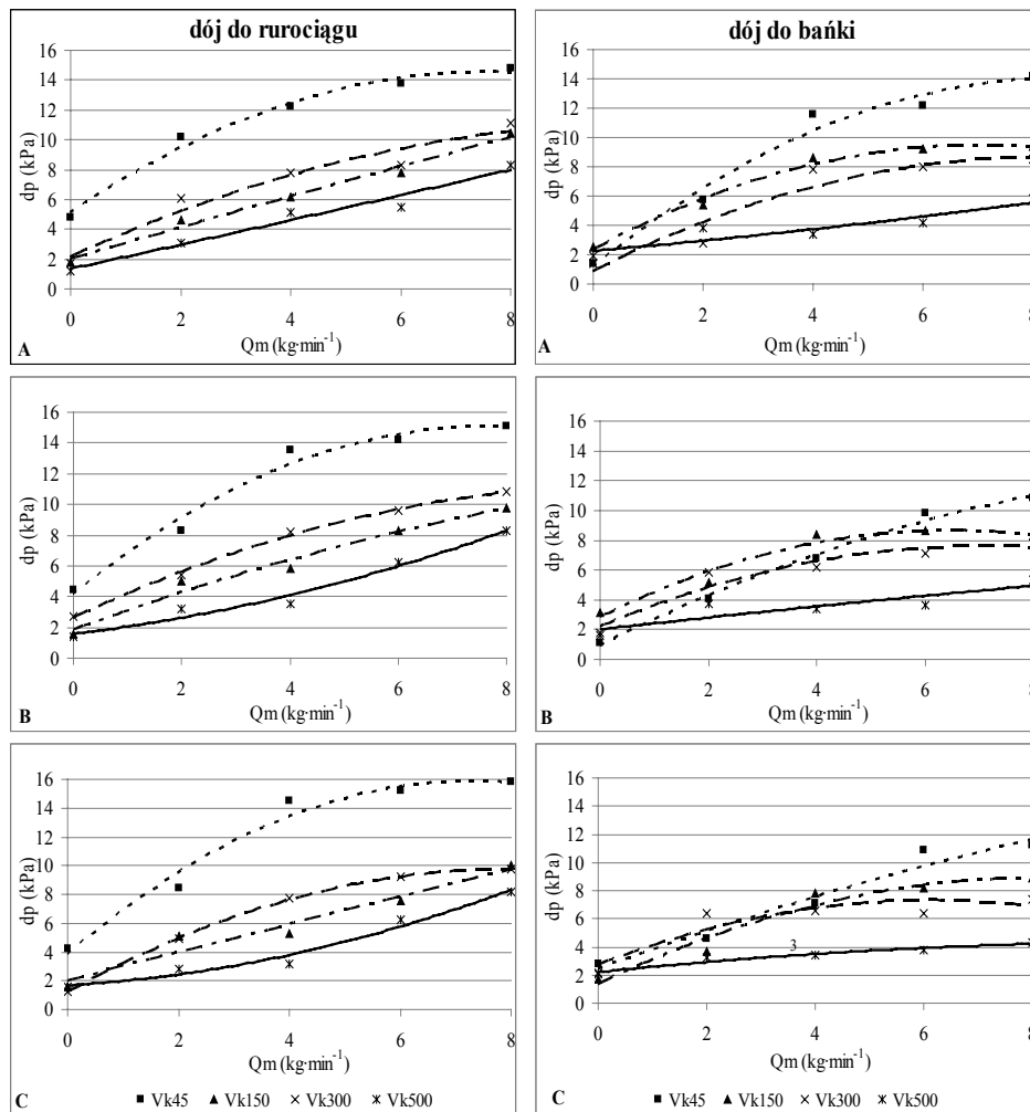
Rysunek 2. Wpływ natężenia strumienia masy cieczy Q_m na wahania podciśnienia w cyklu dp dla zmiennej pojemności komory mlecznej kolektora V_k podczas doju do rurociągu i do bańki przy podciśnieniu systemowym: A – 44 kPa, B – 46 kPa, C – 48 kPa
